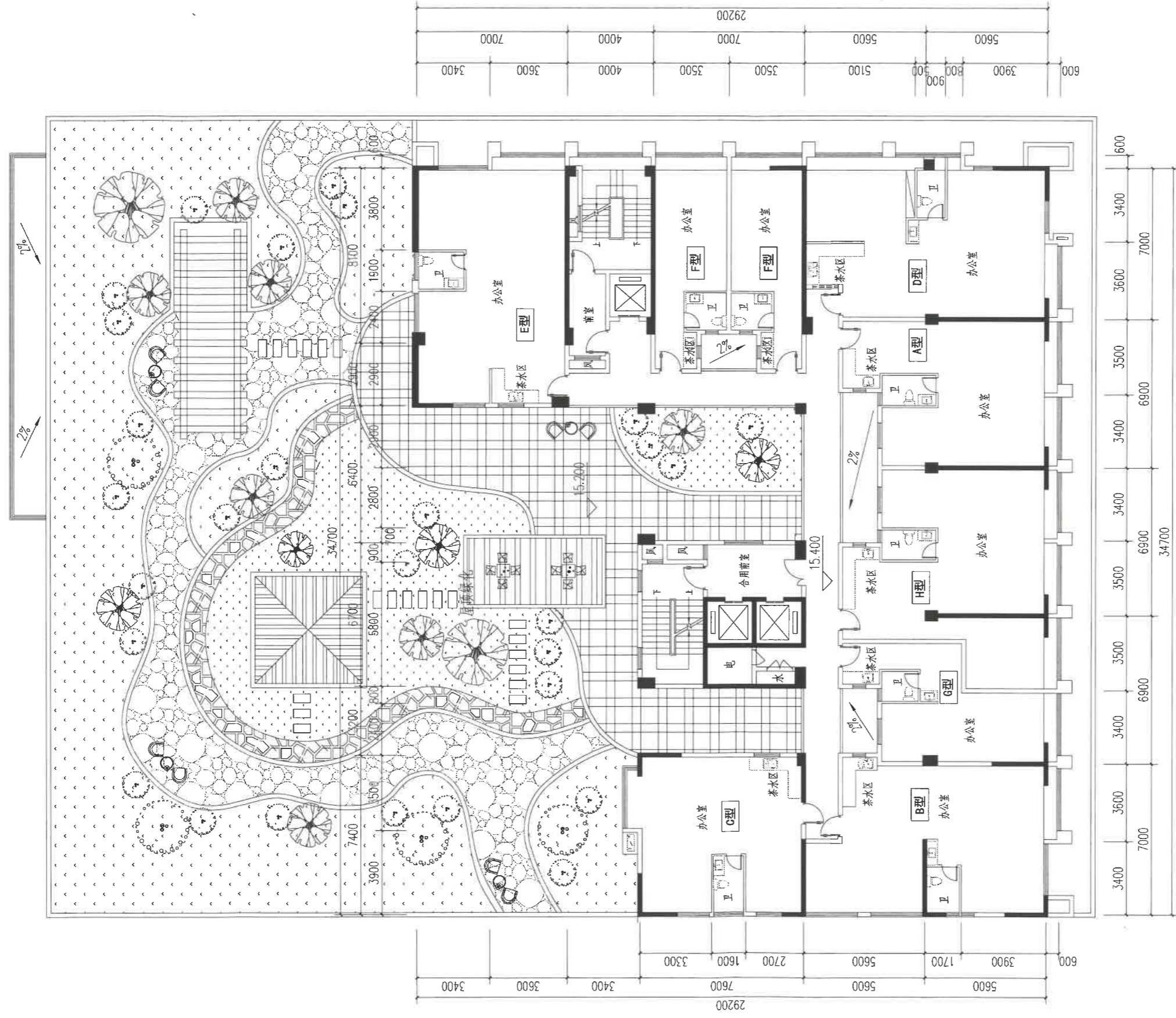
四层平面图
