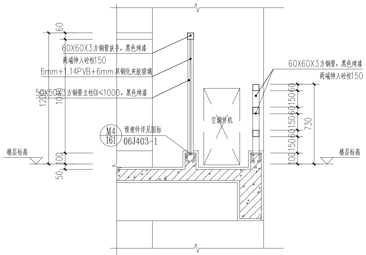
空调栏杆大样图2 1:20
