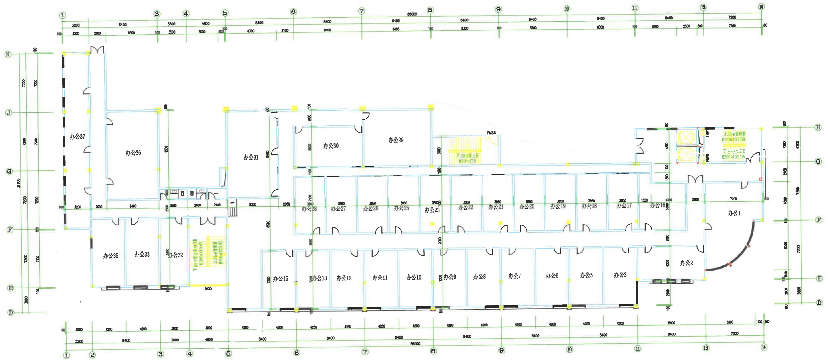
楼座层平面布置图
