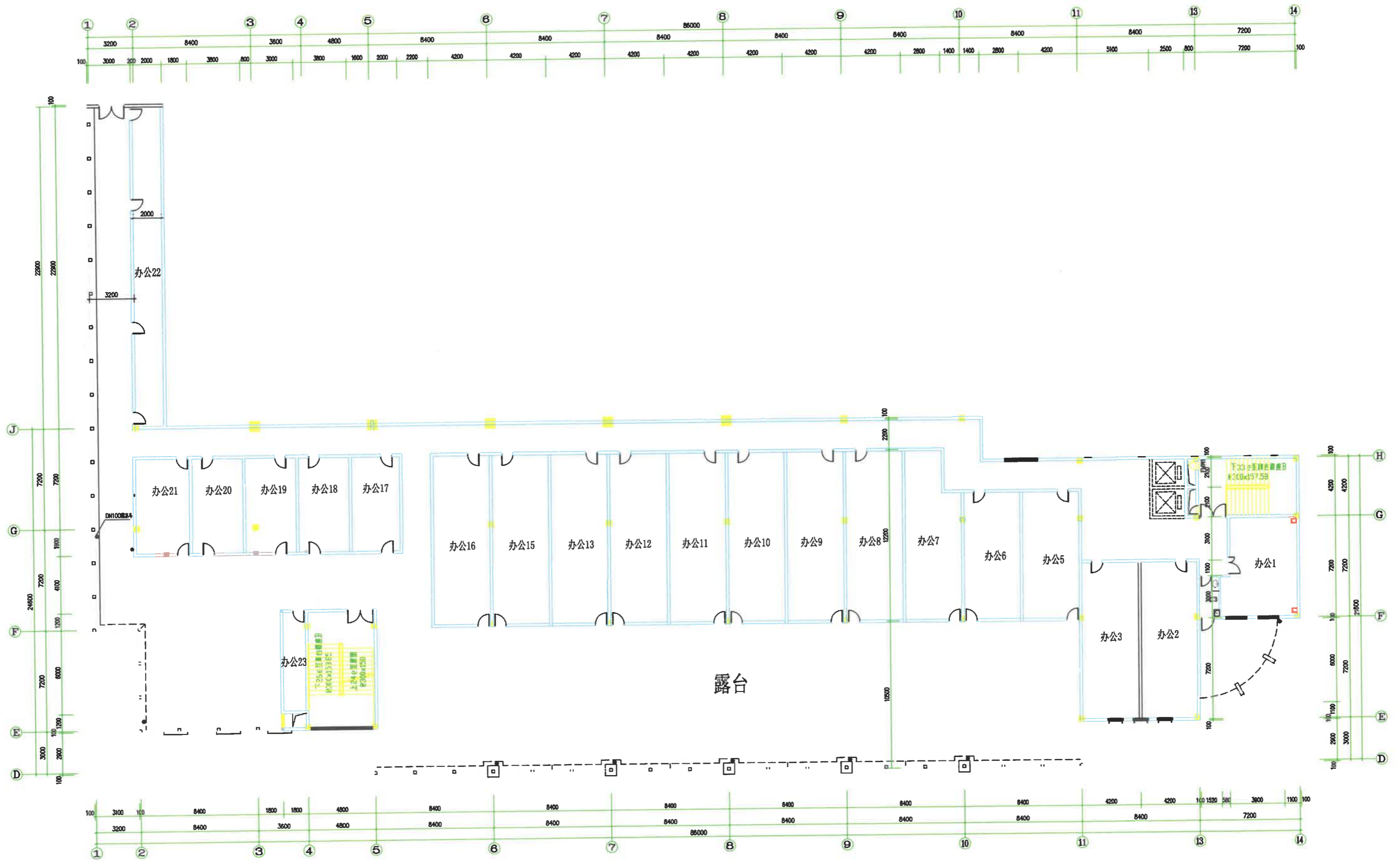
四层平面布置图
