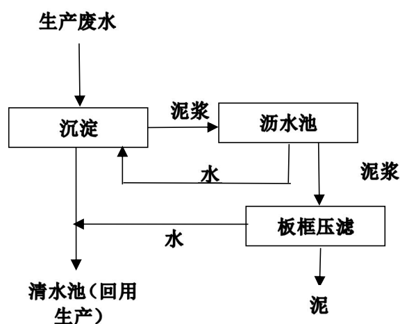
图 4-2 废水处理工艺流程图
